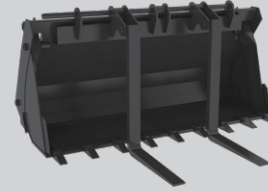
Açılır yükleyici kova uyumlu forklift aparatı
